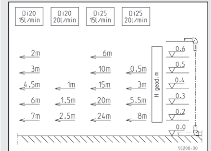
Höhen-/Weitendiagramm
