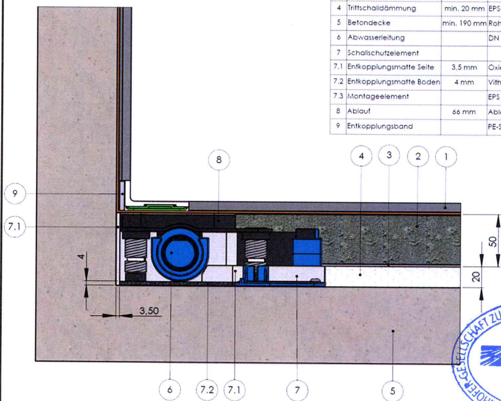
Schnittzeichnung des Prüfaufbaus
