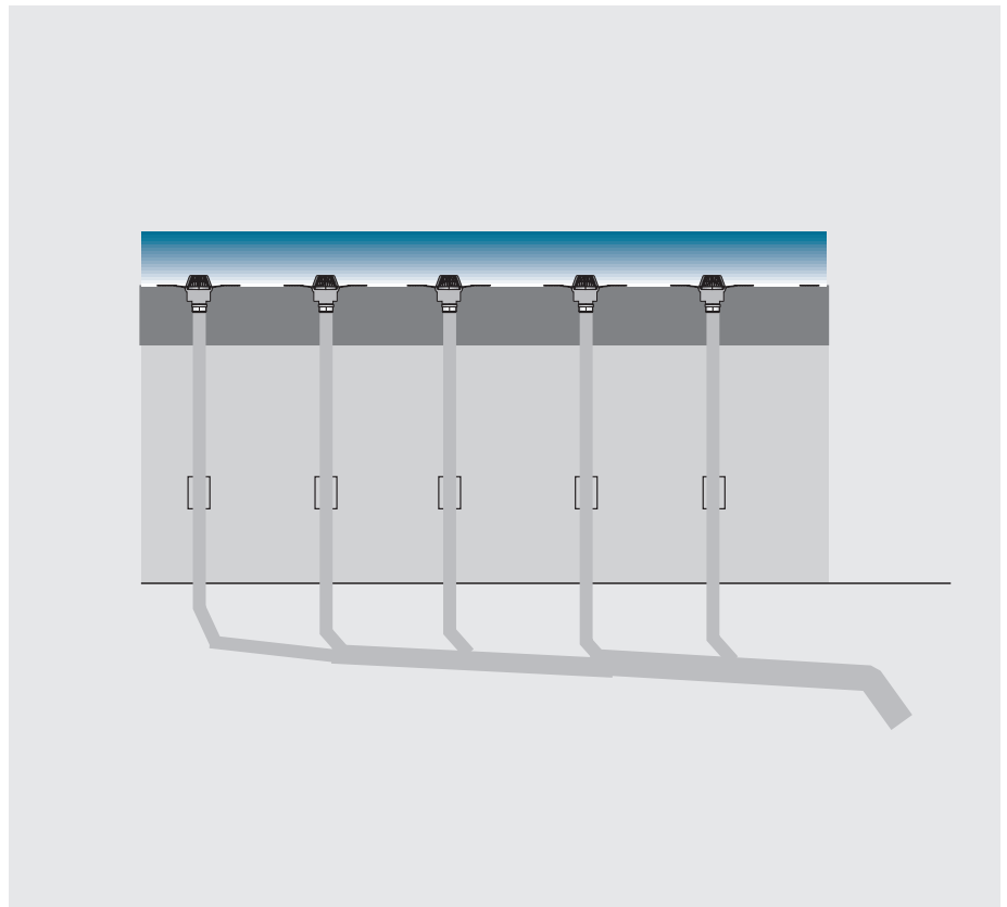
Freispiegelentwässerung
