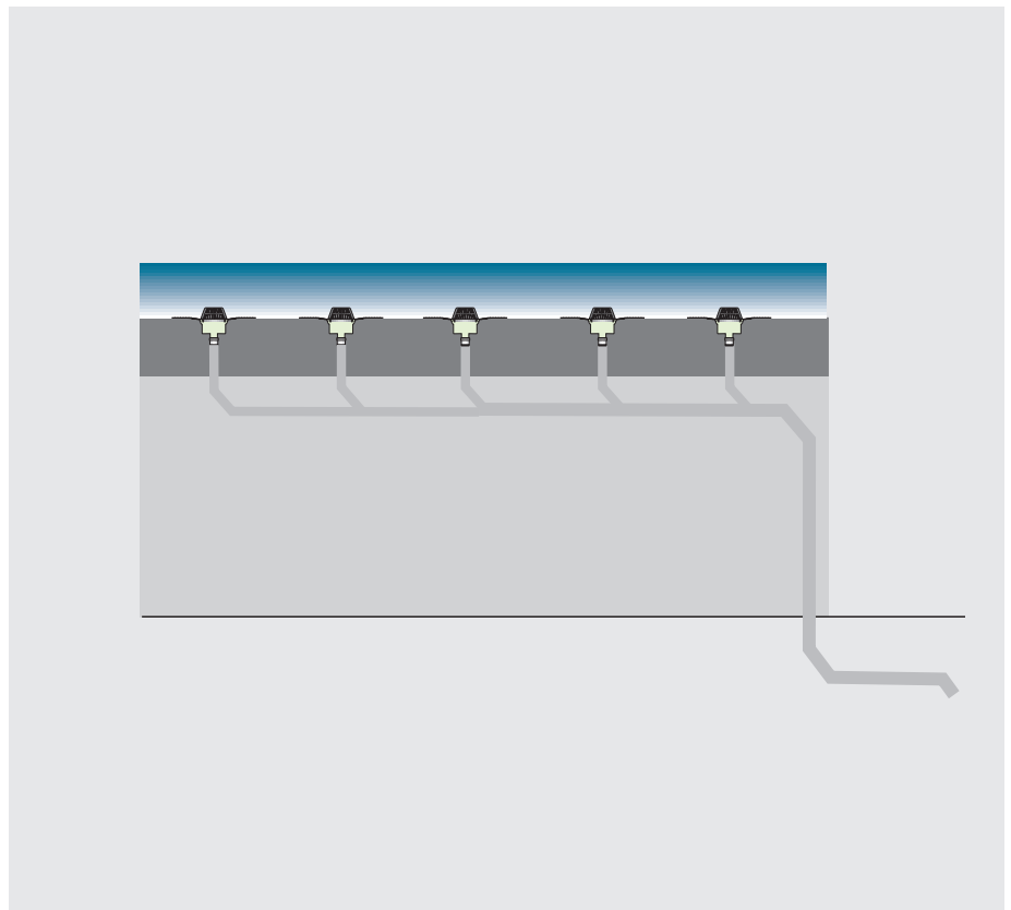
Druckstromentwässerung
